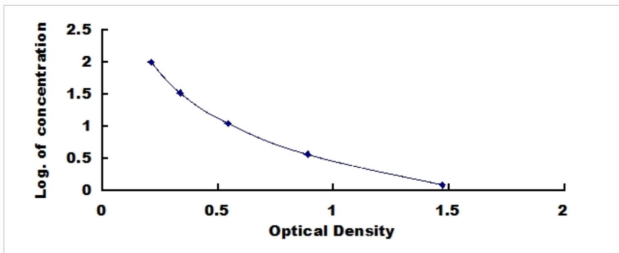
人氧化低密度脂蛋白 (OxLDL) 检测试剂盒标准曲线
