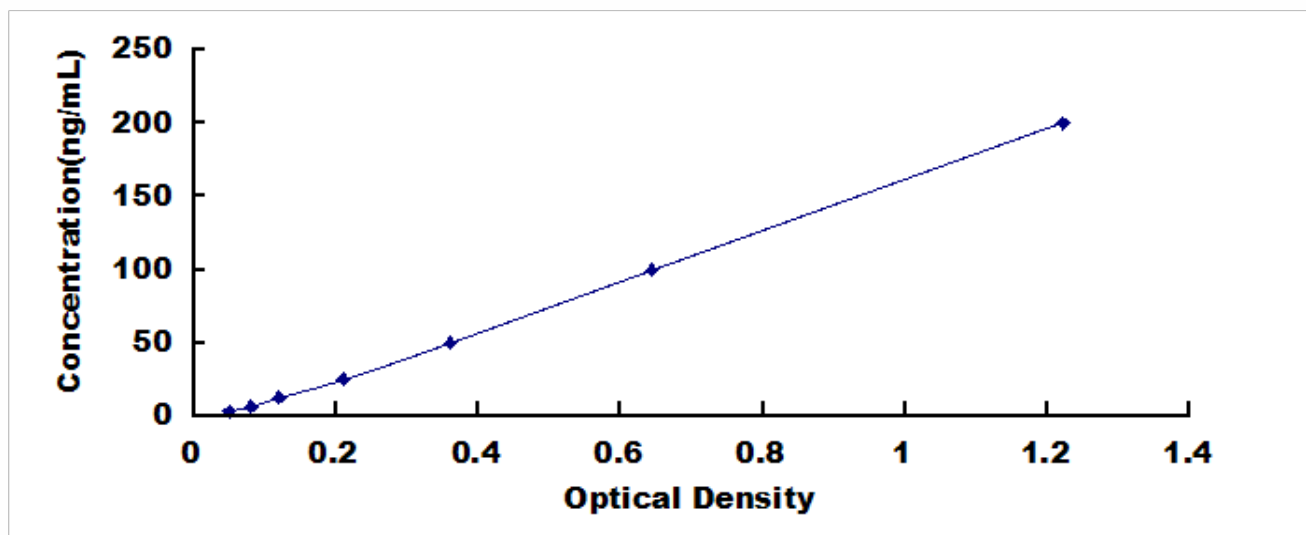
人对氧磷酶 1 (PON1) 检测试剂盒标准曲线
