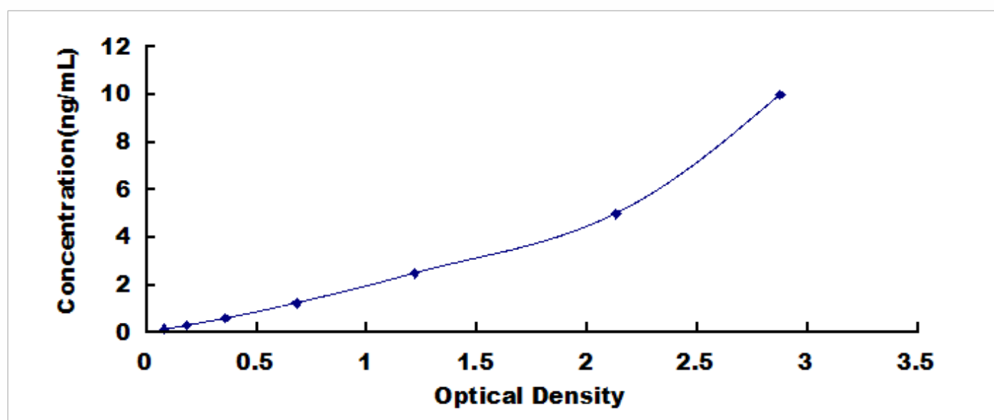
人过氧化还原酶 2 (PRDX2) 检测试剂盒标准曲线
