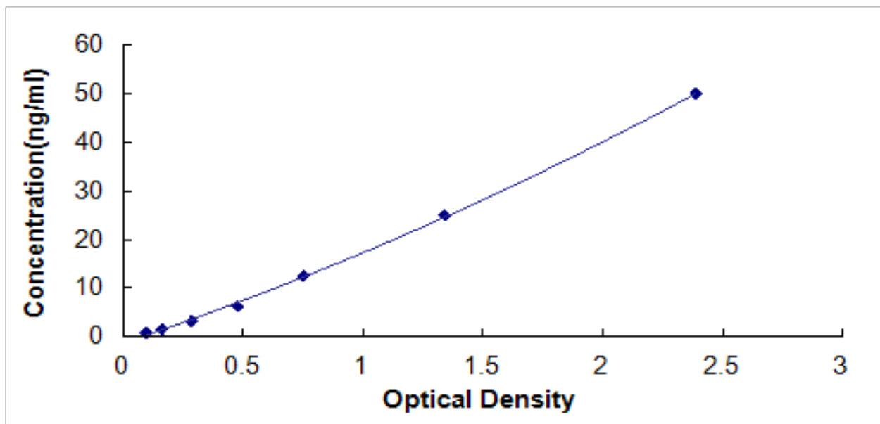
人过氧化物酶体增殖物激活受体 \gamma (PPAR \gamma ) 检测试剂盒标准曲线
