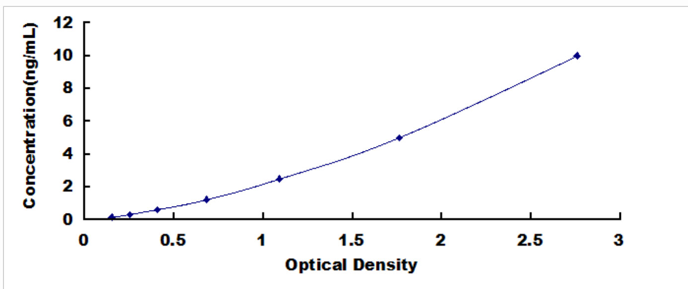
大鼠过氧化物酶体增殖物激活受体 \gamma (PPAR \gamma ) 检测试剂盒标准曲线
