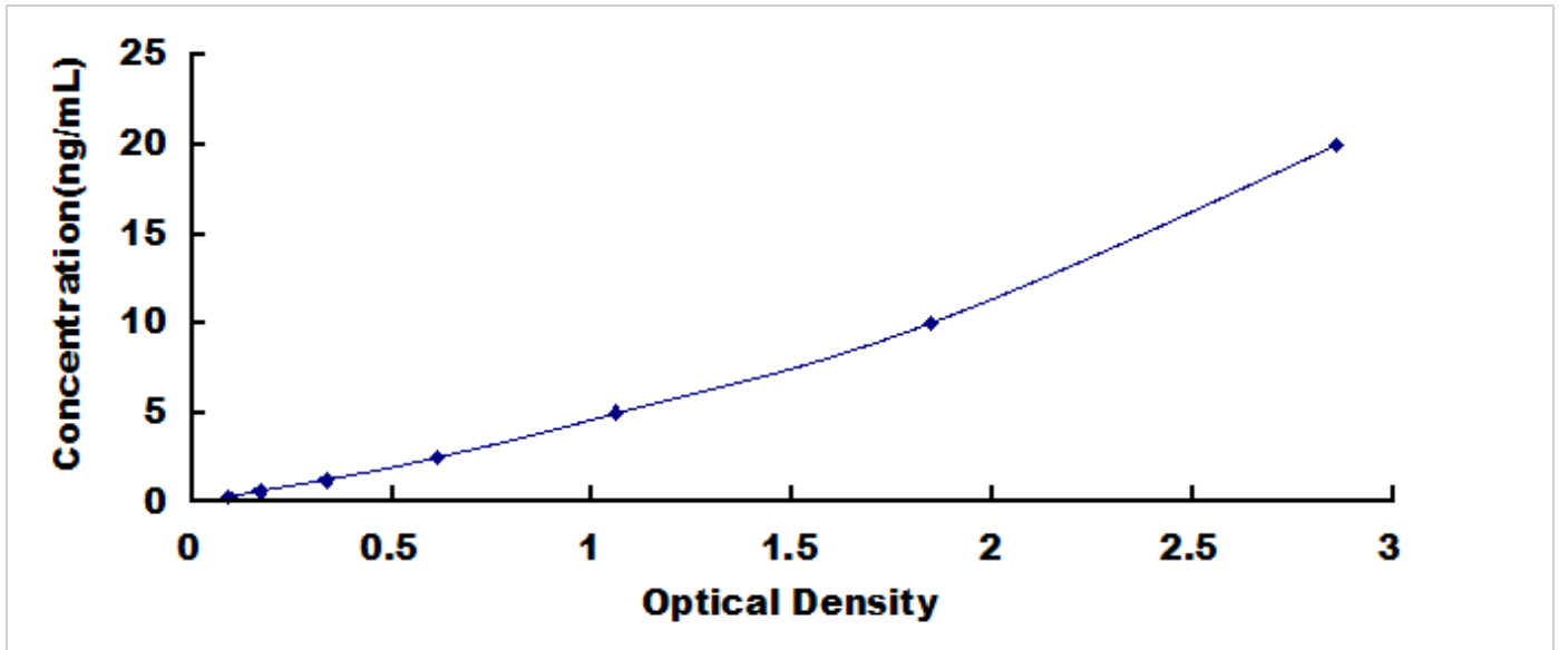
大鼠过氧化物酶体增殖物激活受体 \gamma 辅激活因子 1 \alpha (PPAR \gamma C1 \alpha ) 检测试剂盒标准曲线
