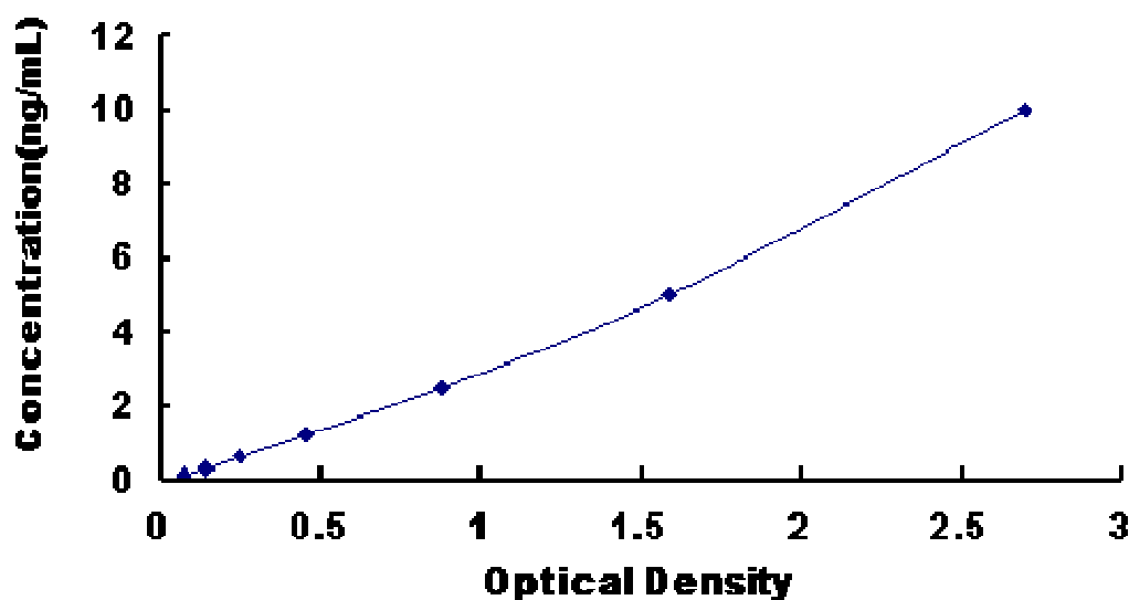
小鼠磷酸肌醇 3 激酶 2 \alpha (PI3K2a) 试剂盒标准曲线
