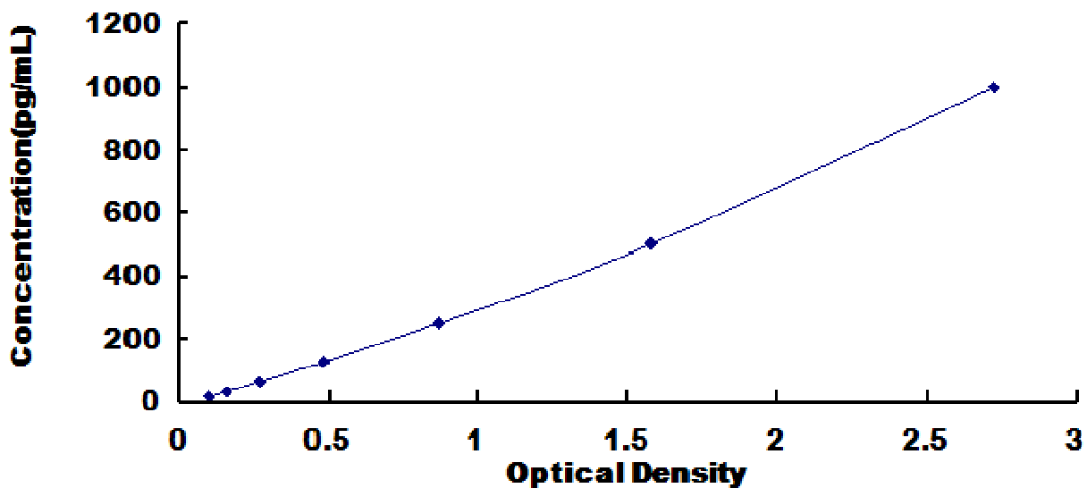
人尿激酶型纤溶酶原激活因子 (uPA) 检测试剂盒标准曲线
