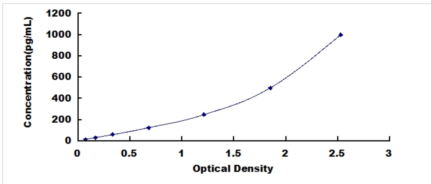
人尿激酶型纤溶酶原激活因子(uPA)检测试剂盒标准曲线
