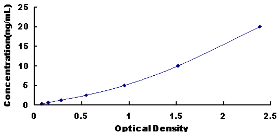
图 1: 大鼠血小板活化因子(PAF)试剂盒标准曲线
