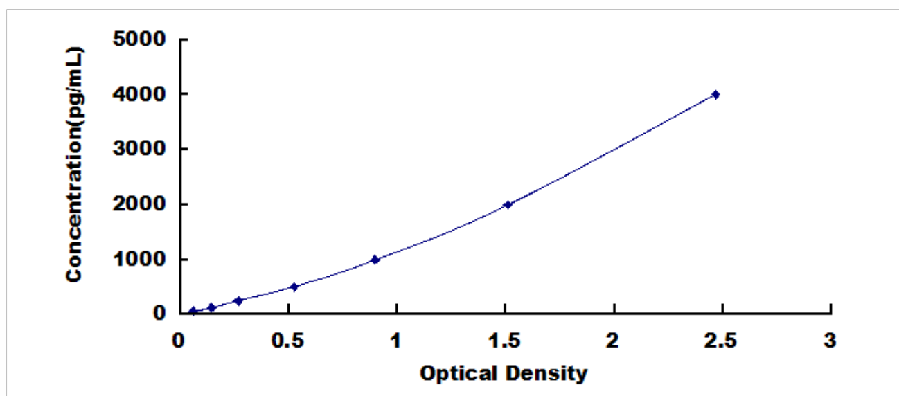
人血小板衍生生长因子 BB (PDGFBB) 检测试剂盒标准曲线
