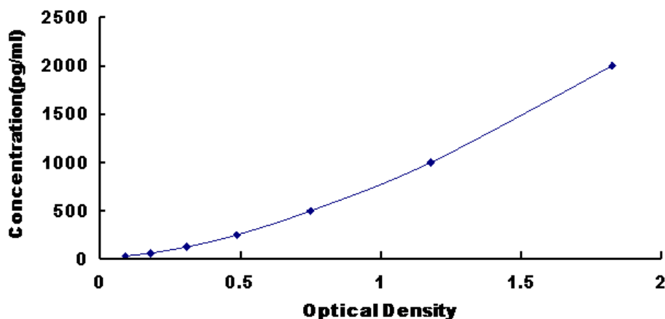
图 1: 人的血小板衍生生长因子 D(PDGF-D)试剂盒标准曲线
