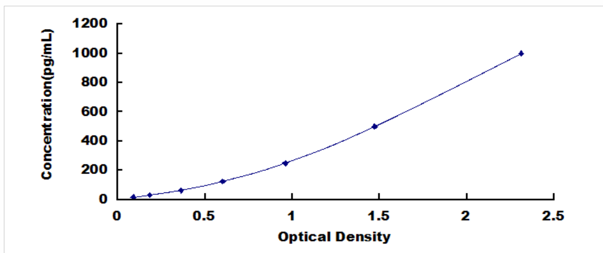
人血小板衍生生长因子 B (PDGFB) 检测试剂盒标准曲线
