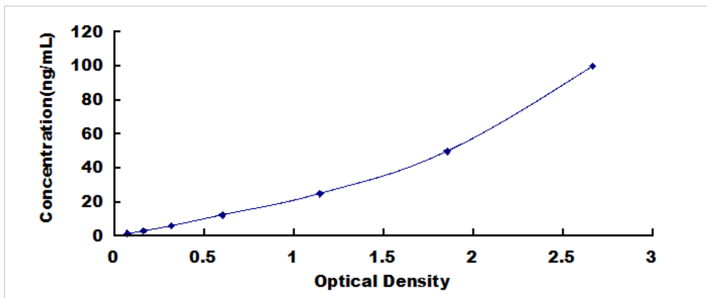
大鼠足孟蛋白 (PCX) 检测试剂盒标准曲线
