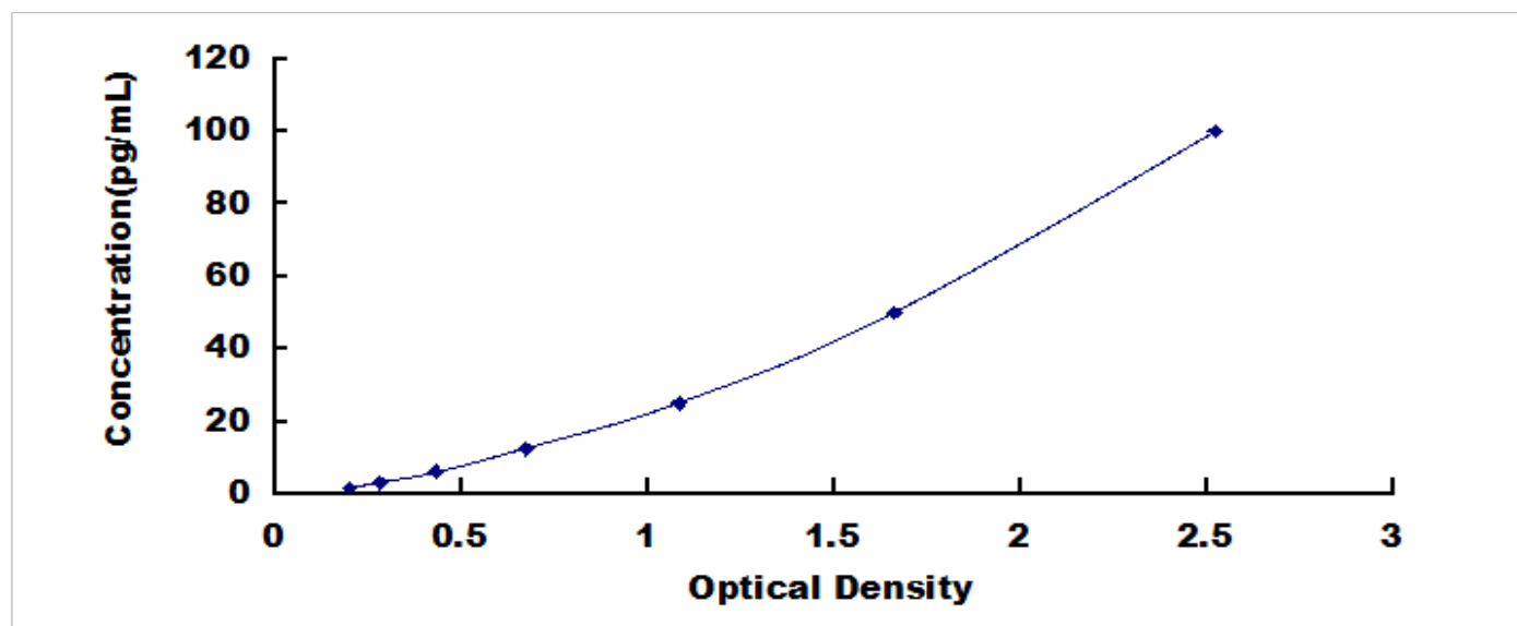
小鼠降钙素原(PCT)检测试剂盒标准曲线
