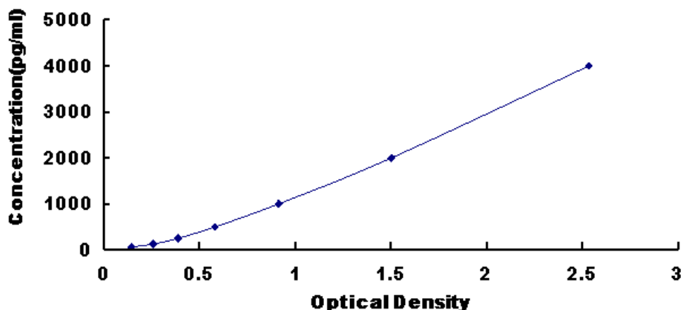
图 1: 大鼠 I 型前胶原(PC- I )试剂盒标准曲线
