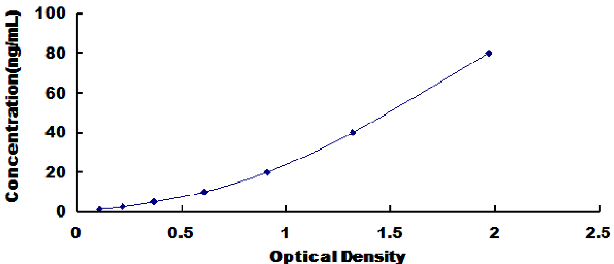
大鼠 I 型前胶原羧基端原肽(P I C P)试剂盒标准曲线
