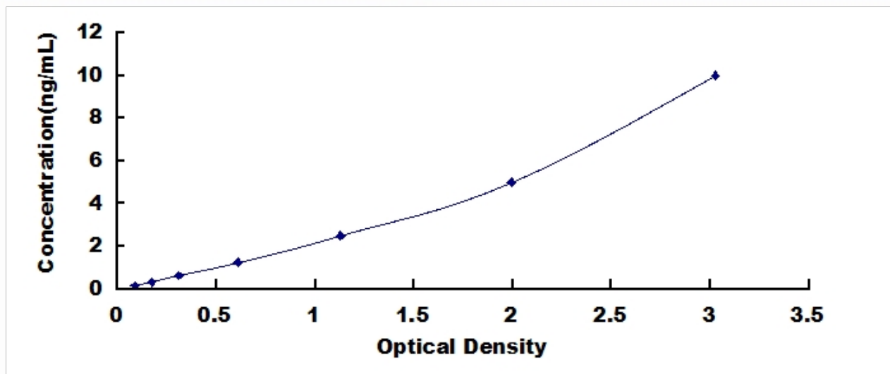
小鼠Ⅲ型前胶原 (PCIII) 检测试剂盒标准曲线
