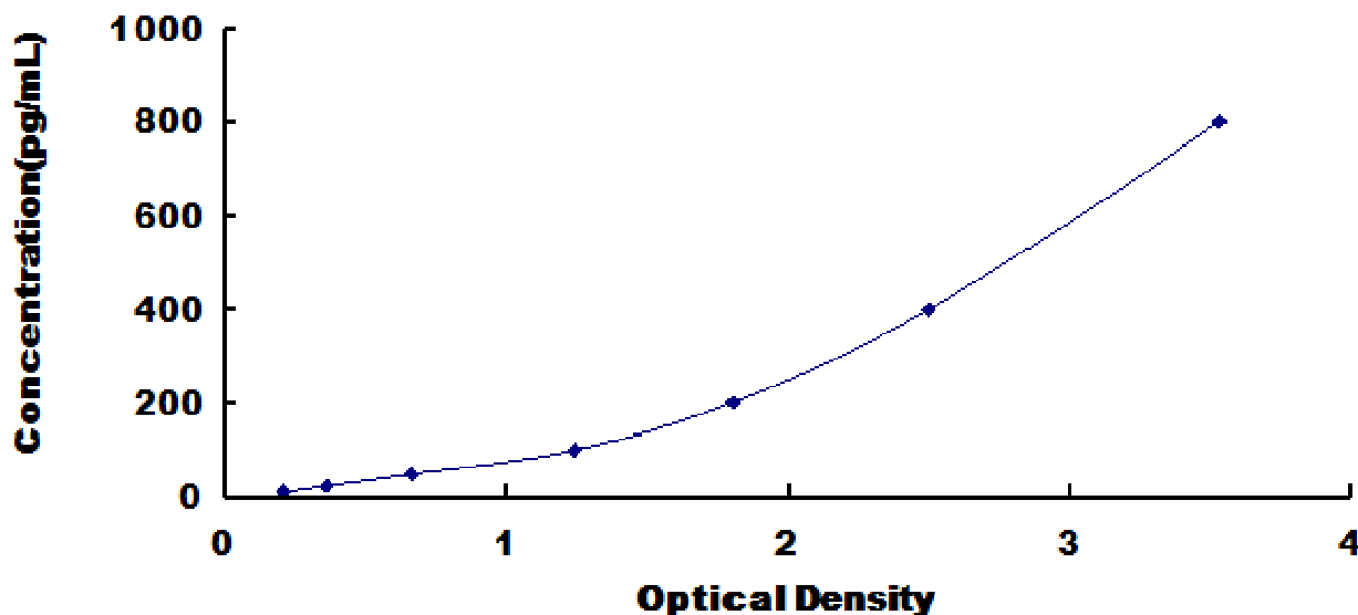
人胰岛素原 (PI) 检测试剂盒标准曲线
