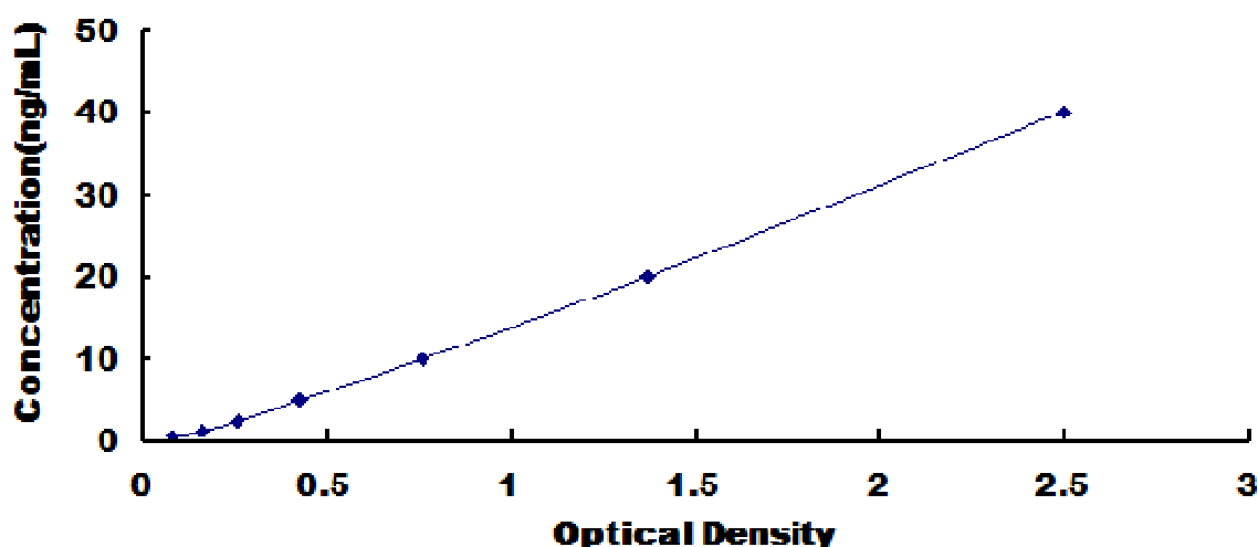
大鼠环加氧酶 1 (PTGS1) 检测试剂盒标准曲线
