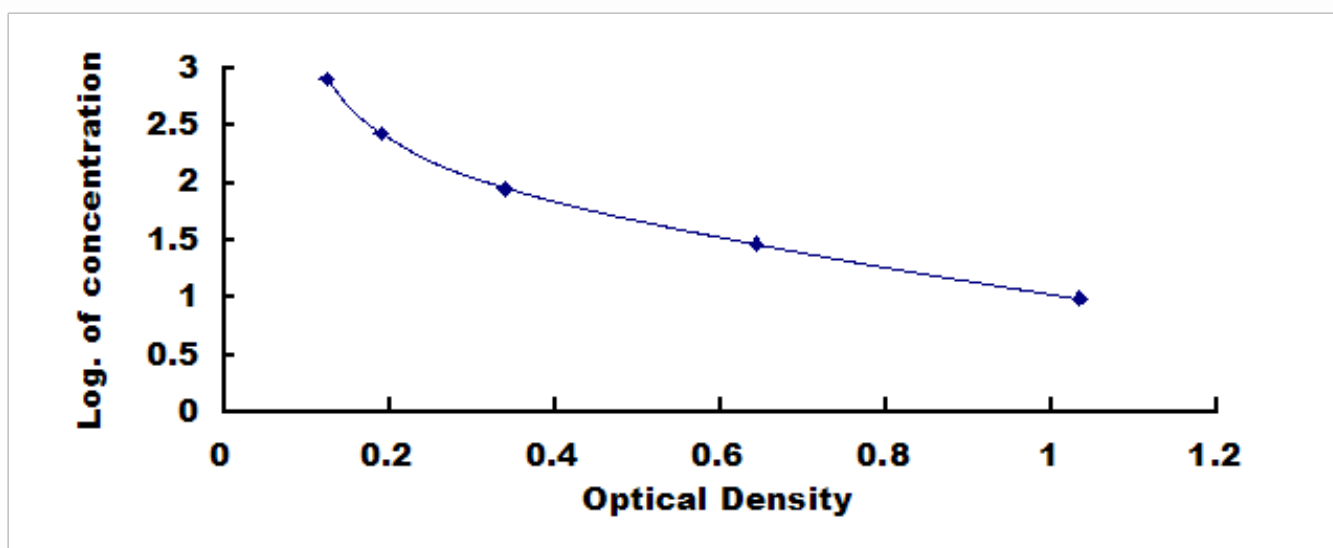
前列腺素 F2 \alpha (PGF2 \alpha ) 检测试剂盒标准曲线
