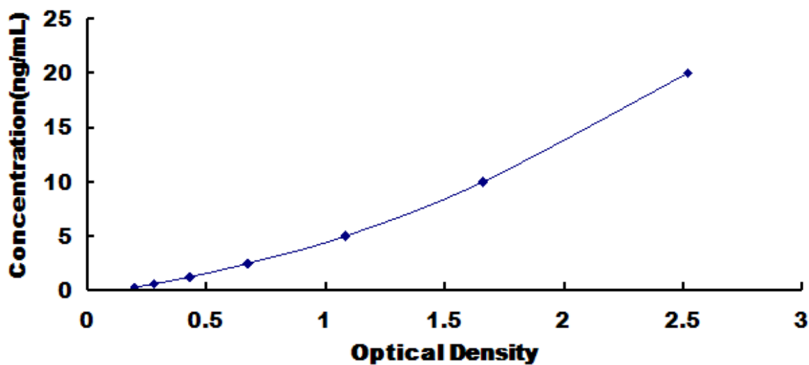
人蛋白酶激活受体 4(PAR4)试剂盒标准曲线
