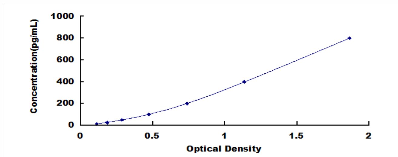
人保护素 (CD59) 检测试剂盒标准曲线
