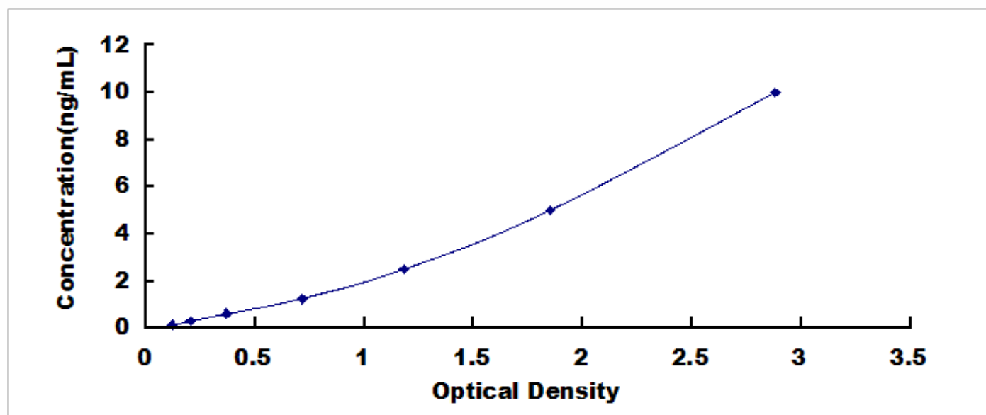
大鼠蛋白激酶 C \epsilon (PKC \epsilon ) 检测试剂盒标准曲线
