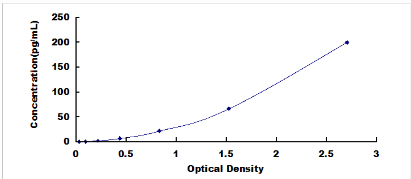
人凝血酶原片段 F1+2 (F1+2) 检测试剂盒标准曲线
