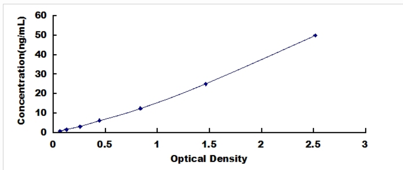
人 M2-型丙酮酸激酶(PKM2)检测试剂盒标准曲线
