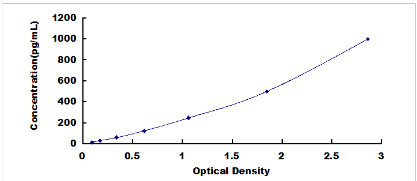
人 R-脊椎蛋白 1 (RSP01) 检测试剂盒标准曲线
