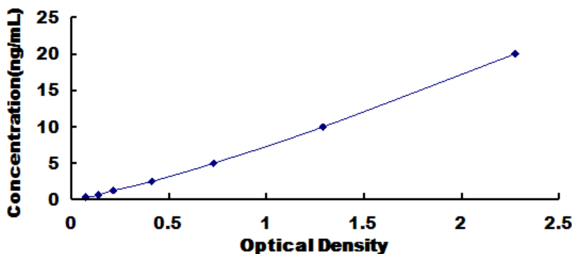
人 RAS 癌基因家族成员，RAB37（RAB37）试剂盒标准曲线
