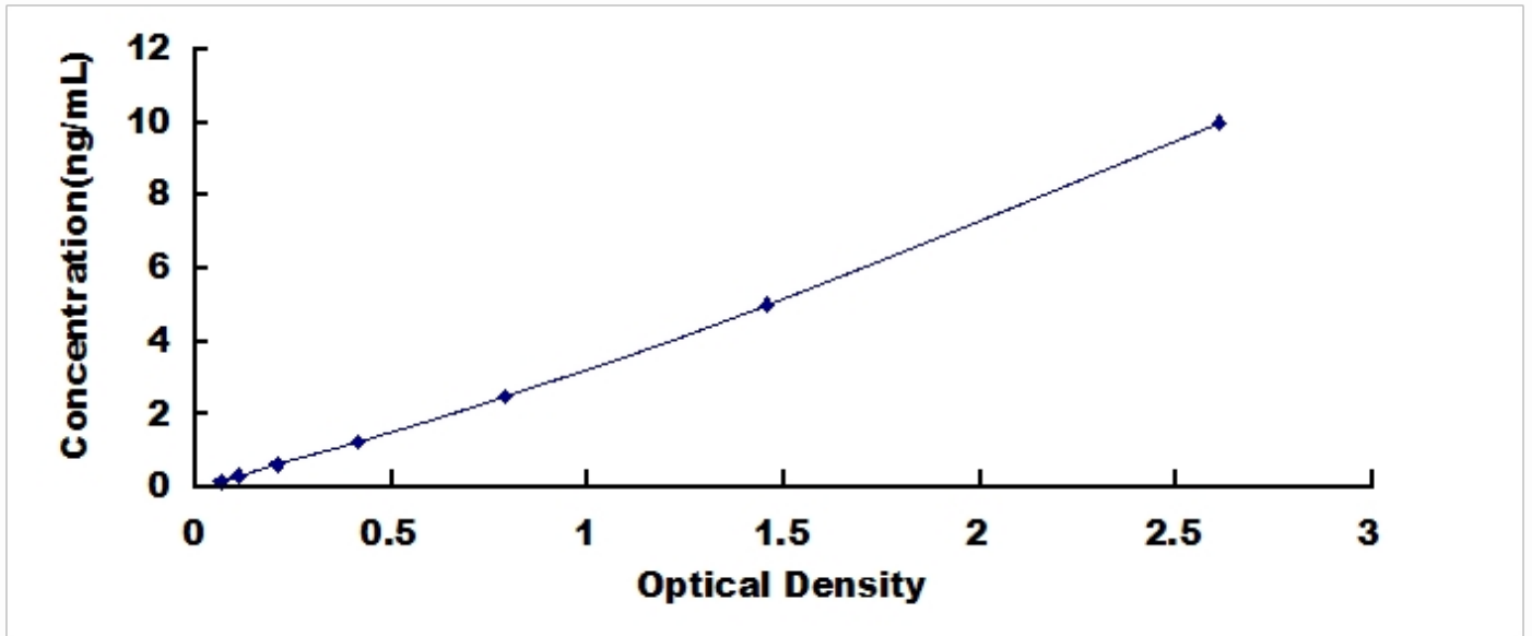
人 Ras 同源基因家族成员 A (RHOA) 检测试剂盒标准曲线
