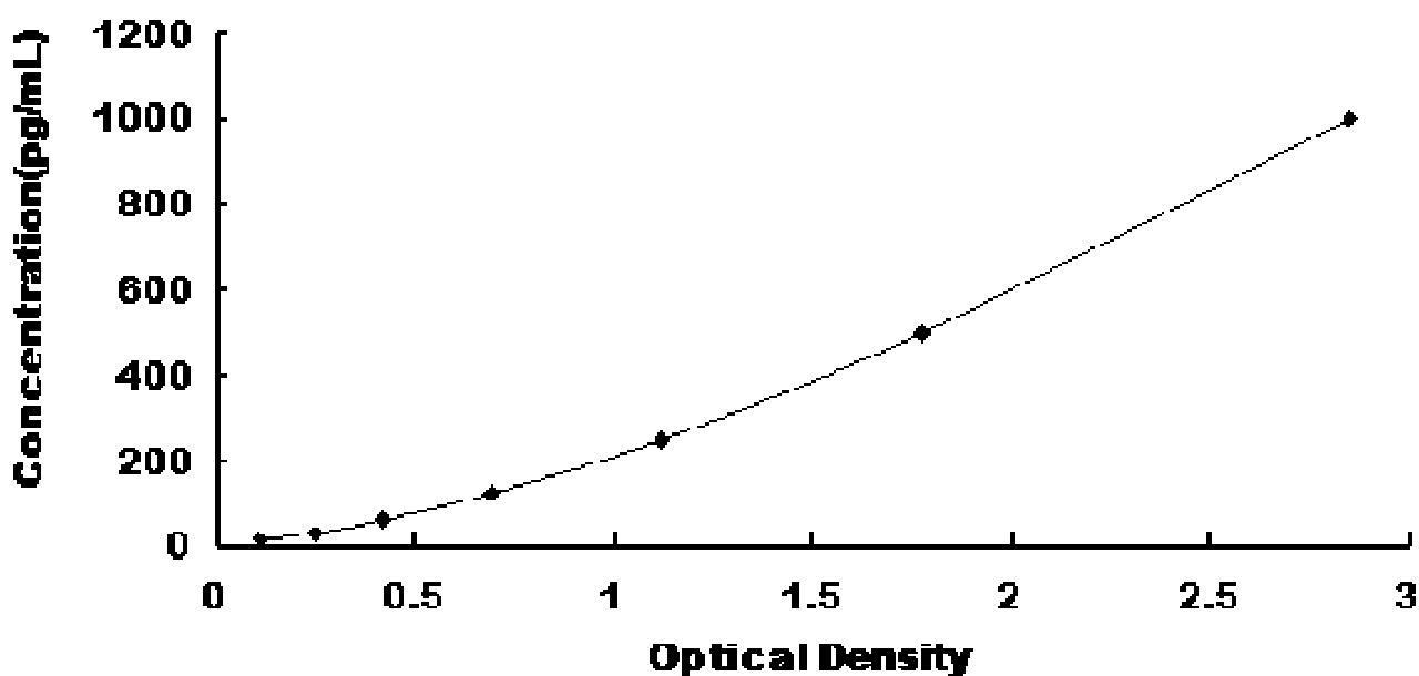
人络丝蛋白(RL)试剂盒标准曲线
