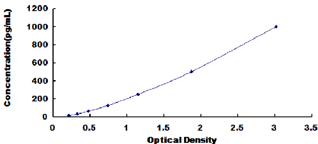
大鼠络丝蛋白(RL)试剂盒标准曲线
