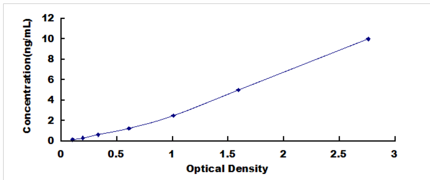
人再生胰岛衍生蛋白 4(REG4)检测试剂盒标准曲线
