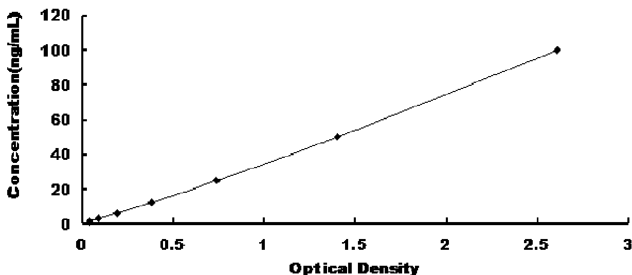
大鼠 S11 钙结合蛋白(S100A11)试剂盒标准曲线
