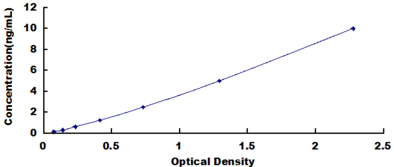
小鼠 SPARC 相关组件钙结合蛋白 1 (SMOC1) 检测试剂盒标准曲线
