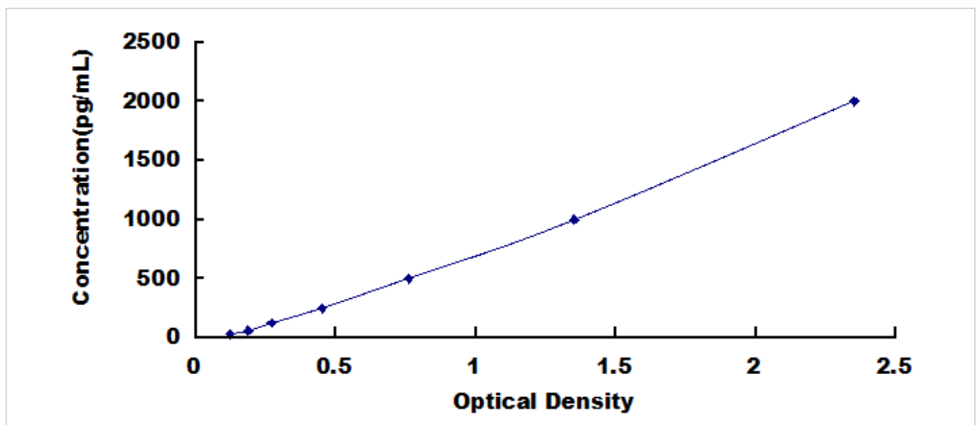
大鼠分泌型卷曲相关蛋白 4 (SFRP4) 检测试剂盒标准曲线
