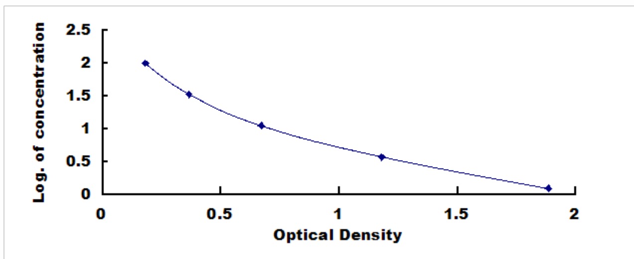
猪分泌型免疫球蛋白 A(sIgA) 检测试剂盒标准曲线
