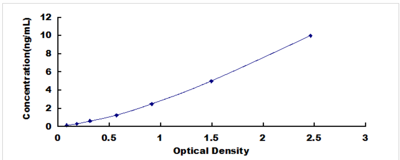
大鼠信号素 3A (SEMA3A) 检测试剂盒标准曲线
