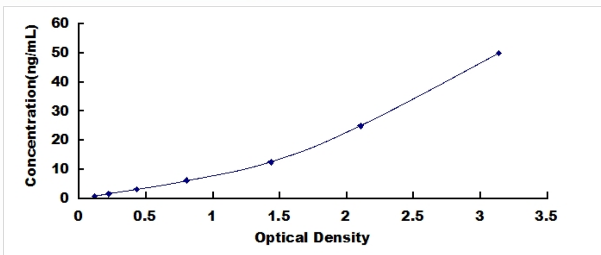
人信号素 5A (SEMA5A) 检测试剂盒标准曲线
