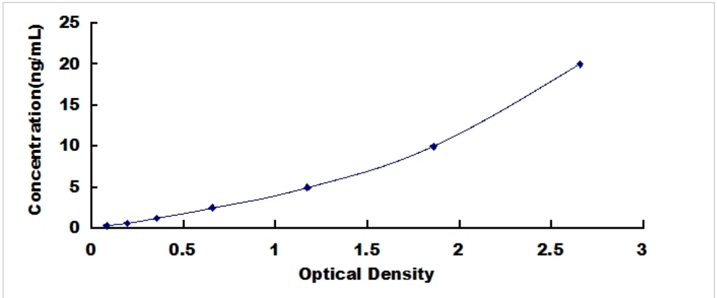
人胞裂蛋白 5 (SEPT5) 检测试剂盒标准曲线
