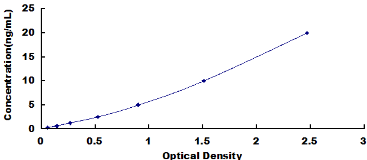
人死骨片 1 (SQSTM1) 检测试剂盒标准曲线
