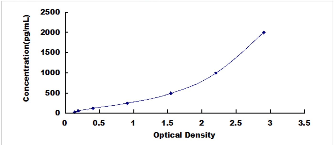
人 5-羟色胺转运蛋白 (SERT) 检测试剂盒标准曲线
