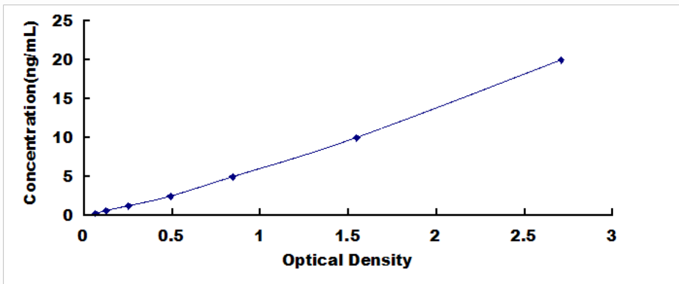
人性别决定区 Y 框蛋白 9 (SOX9) 检测试剂盒标准曲线
