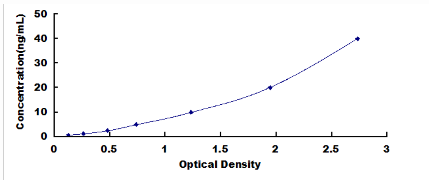
大鼠性激素结合球蛋白 (SHBG) 检测试剂盒标准曲线
