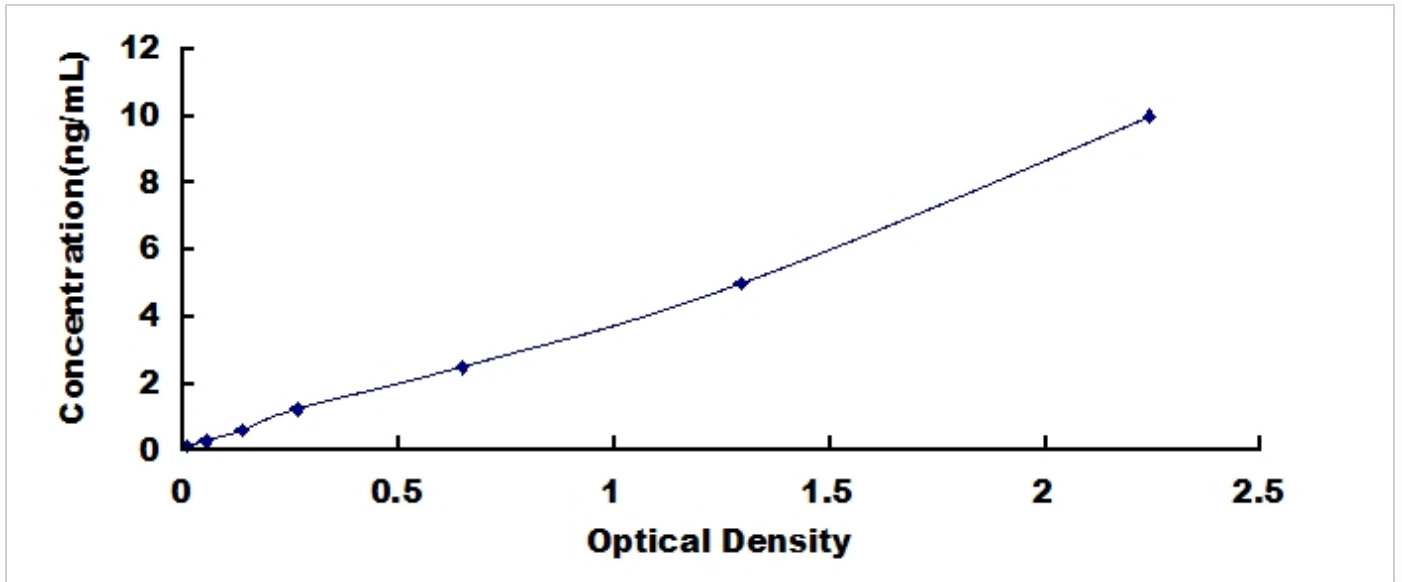
人 Snail 同源物 1 (SNAI1) 检测试剂盒标准曲线
