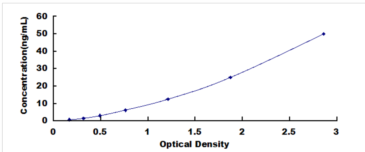
大鼠钠/葡萄糖协同转运蛋白 2 (SGLT2) 检测试剂盒标准曲线
