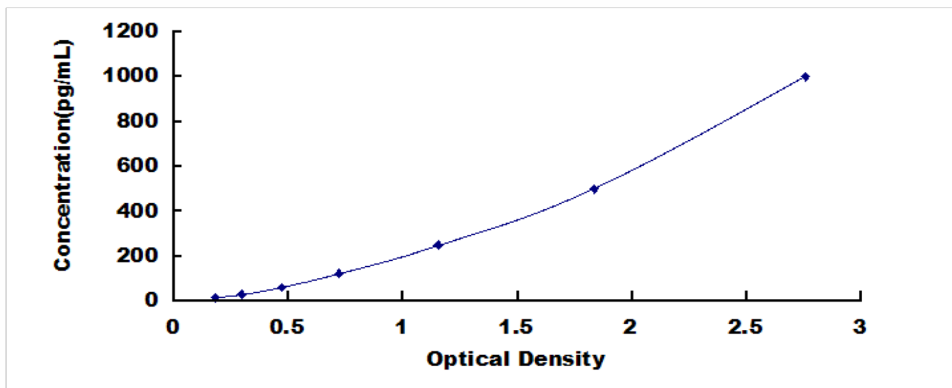
兔超氧化物歧化酶 1 (SOD1) 检测试剂盒标准曲线
