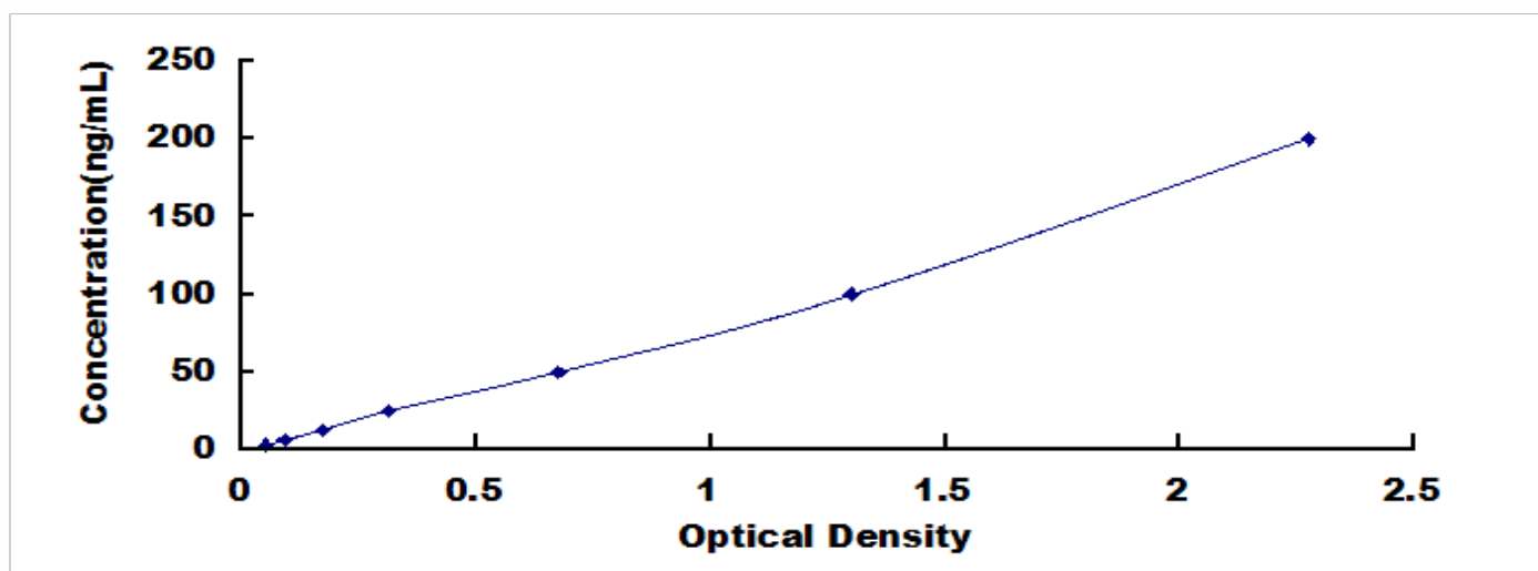
小鼠胞外超氧化物歧化酶(SOD3)检测试剂盒标准曲线
