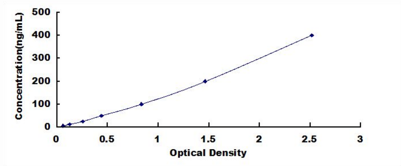
人表面活性物质关联蛋白 D (SPD) 检测试剂盒标准曲线
