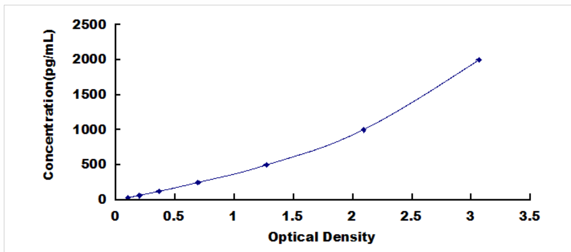
人存活素 (Surv) 检测试剂盒标准曲线
