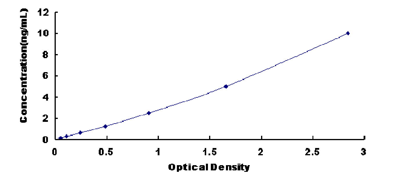
人多配体蛋白聚糖 4(SDC4)试剂盒标准曲线
